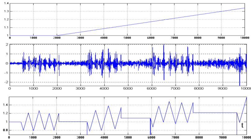
Рисунок 2. Динаміка зміни коефіцієнту передачі моделі ОК за каналом дії контрольованого збурення k_{\text{кгу}} , регульованої змінної y(t) та коефіцієнта k_m при моделювання роботи інваріантної САР і роботи пошукового алгоритму оптимізації.
