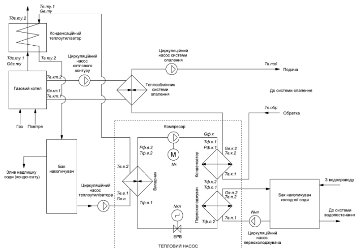
Рисунок 1. Параметризована схема процесу глибокої утилізації тепла з використанням теплового насоса
