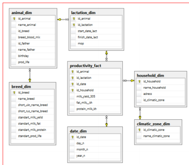
Рис. 2 Структура СД для СПІР щодо реалізації задач селекції у тваринництві
