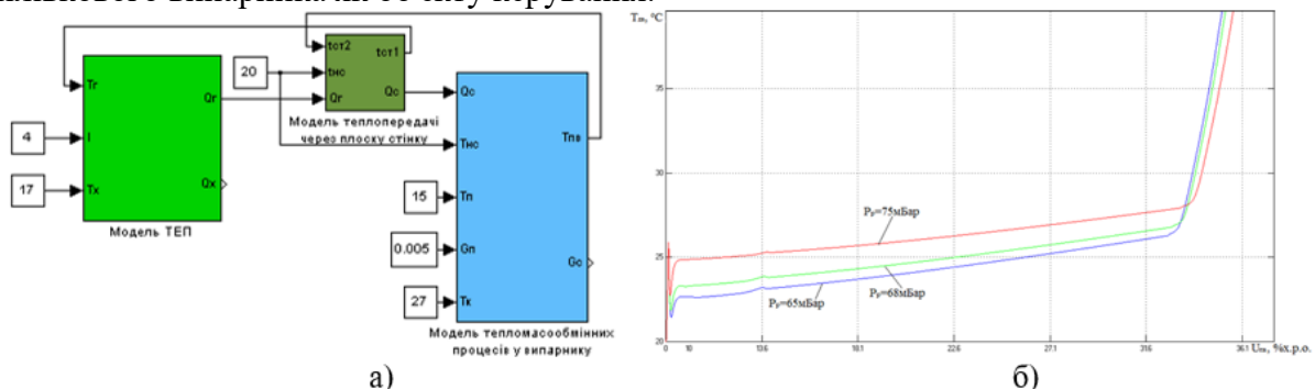
Рисунок 2 – а) реалізація в середовищі Simulink моделі тепломасообмінних процесів у випарнику та математичної моделі термоелектричного плівкового випарника як об'єкту керування; б) квазістатичні залежності температури продукту у випарнику від струму живлення ТЕП при різному тиску в ресивері.
