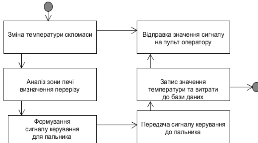
Рисунок 2. Діаграми стану.
