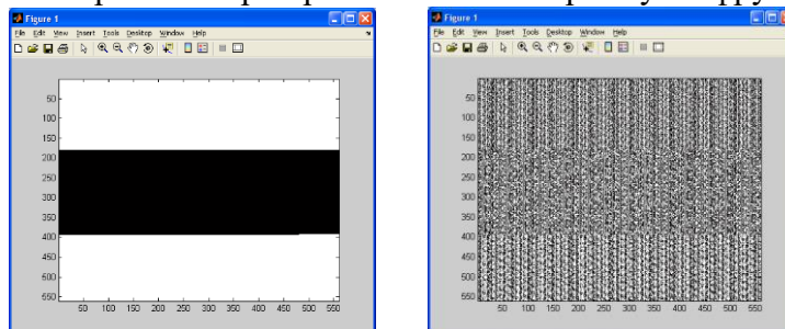
Рис.1 Візуалізація роботи автомата Лоренца в кільці Z(2^8) .
